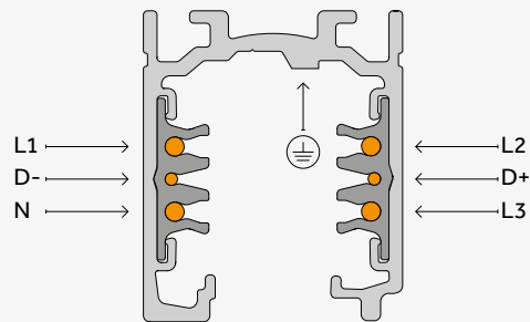
Stromschiene
