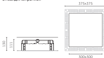
Mit Einputzrahmen/ Сневидимой рамкой
