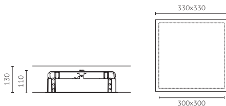
Mit Blendrahmen/ Свидимой рамкой
