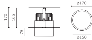
Mit Blendrahmen/ Свидимой рамкой
