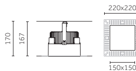
Mit Einputzrahmen/ Сневидимой рамкой
