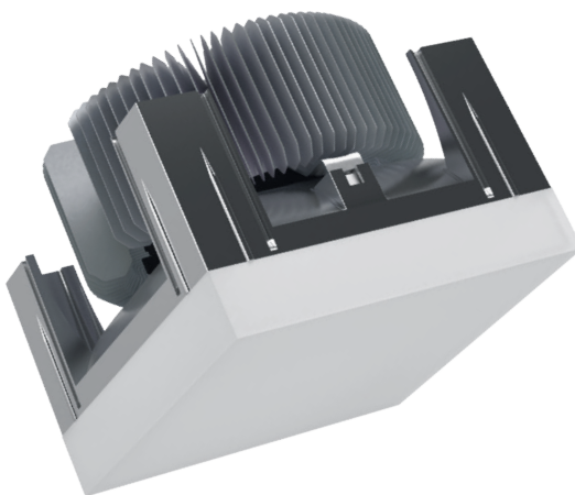
DE Kunststoffabstandshalter für drei Positionen der Abdeckung: eingelassen, bündig abgeschlossen, vorgesetzt. RU Пластиковая прокладка для трех положений диффузора: встроеное, вровень с поверхностью, выступающее
