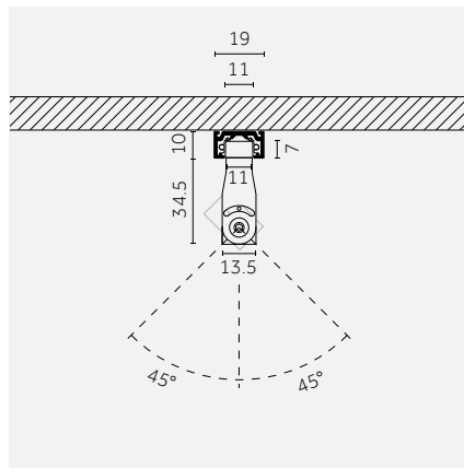
EN +/- 45° adjustability. IT Orientabilità di +/- 45°.
