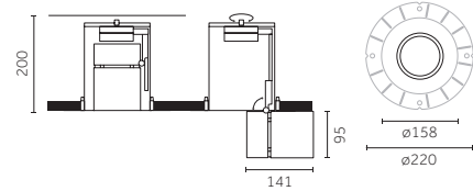
Collettere apparente/ Conaro visibile
