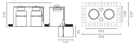
Collerette apparente/ Con aro visibile
