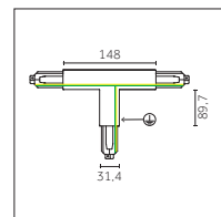
T-connector
