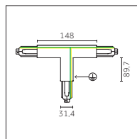
T-connector
