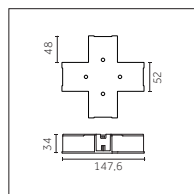
Tapa para unión cruciforme
