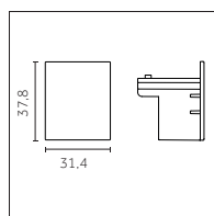
Tapa de cierre para carril de superficie con tornillo de bloqueo
