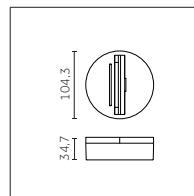
Base para la fijación de techo del adaptador DALI sin el utilizzo del carril
