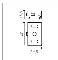
Estribo para fijación de techo
