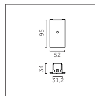
Tapa para cabeza L 95 mm
