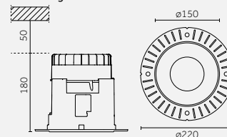
Trimless/ Senza flangia
