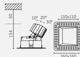
Trimless/ Senza flangia
