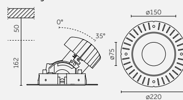
Trimless/ Senza flangia
