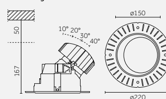
Trimless/ Senza flangia
