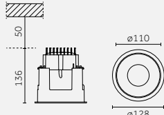
Visible trim/ Con flangia
