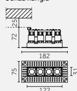
Trimless/ Senza flangia
