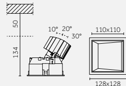
Visible trim/ Con flangia
