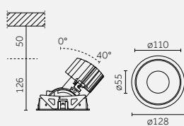
Visible trim/ Con flangia
